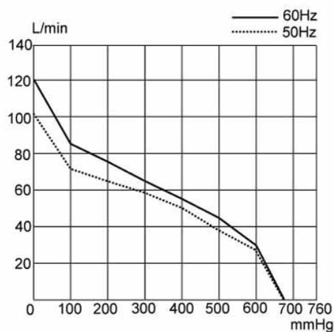
真空曲線表：
